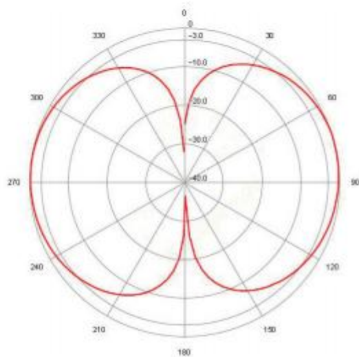
VHF E-PLANE
