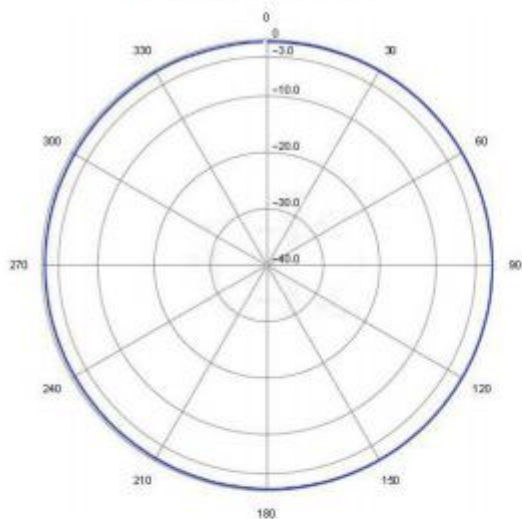
UHF H-PLANE
