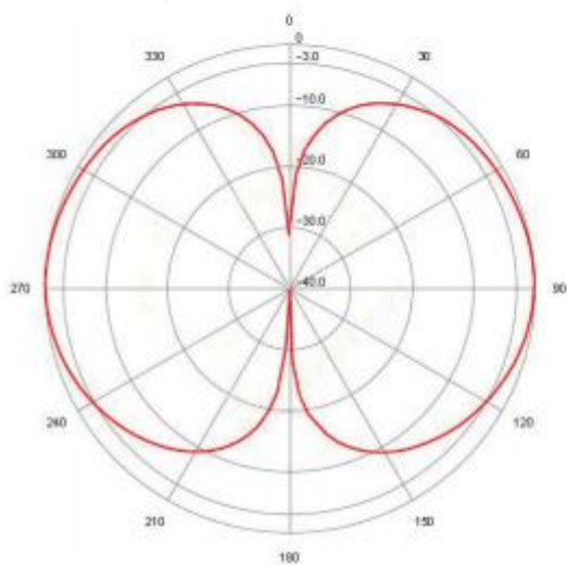
UHF E-PLANE
